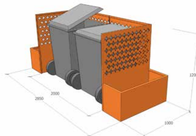
Bild 2: Mått Green City Sopgarage
